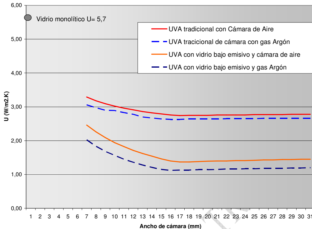
Gráfica 1: Relación entre la transmitancia con el ancho de cámara para distintas UVAs
